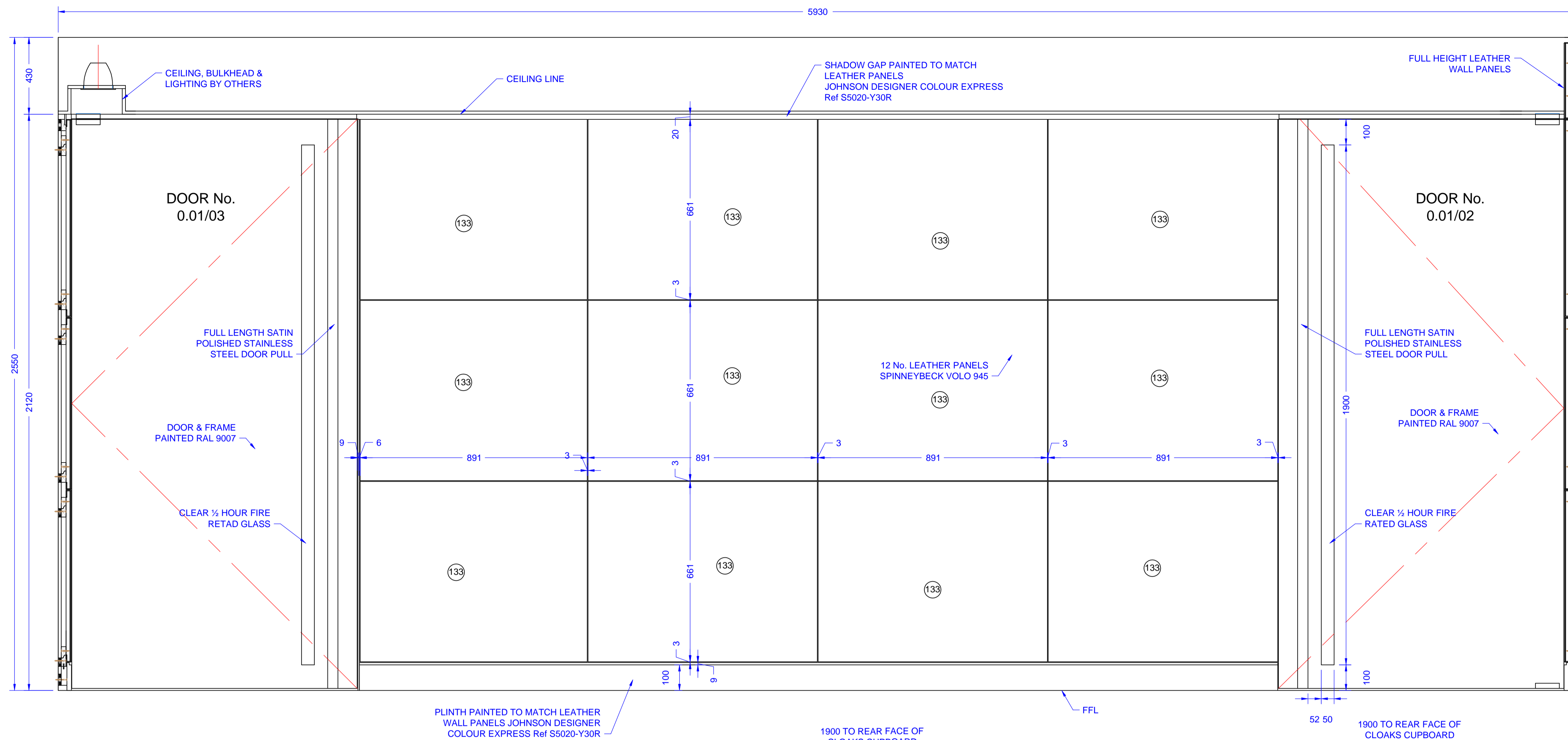
ELEVATION 'C'
