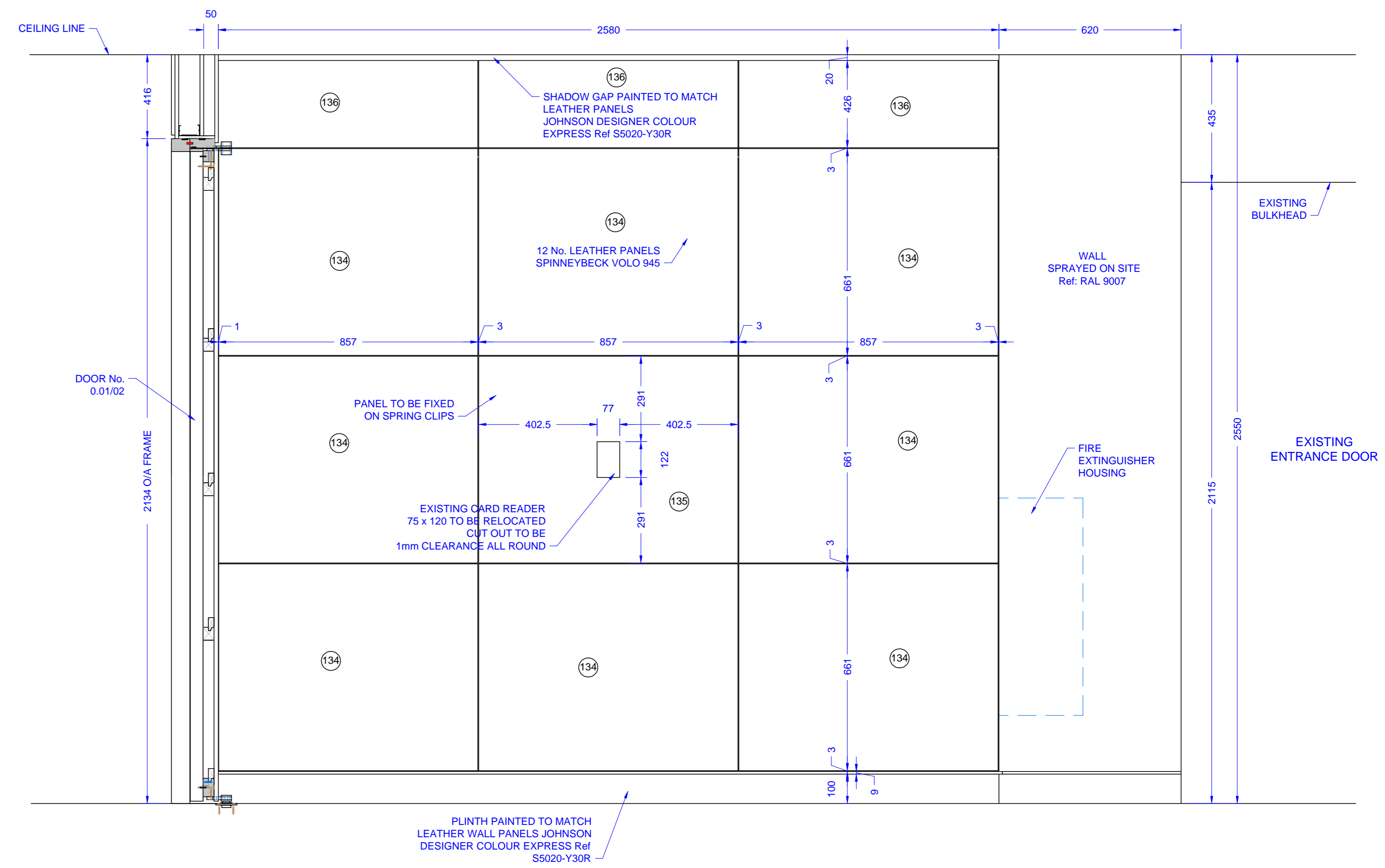
ELEVATION 'D'
